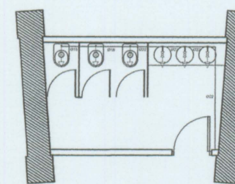
DETALLE ASEO TIPO B
