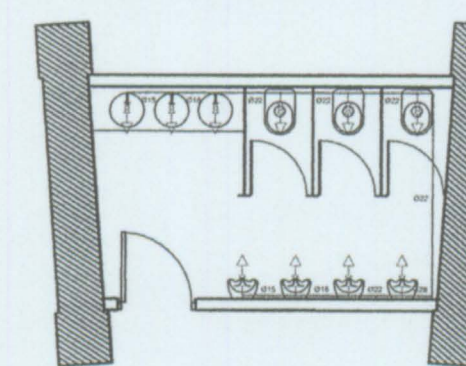
DETALLE ASEO TIPO A
