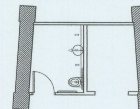
DETALLE ASEO TIPO C
