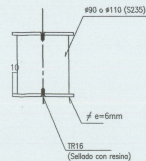
DETALLE PASADOR 1/5
