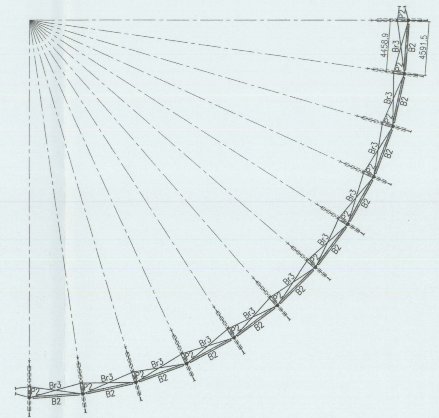
SECCIÓN D-D' 1/200
