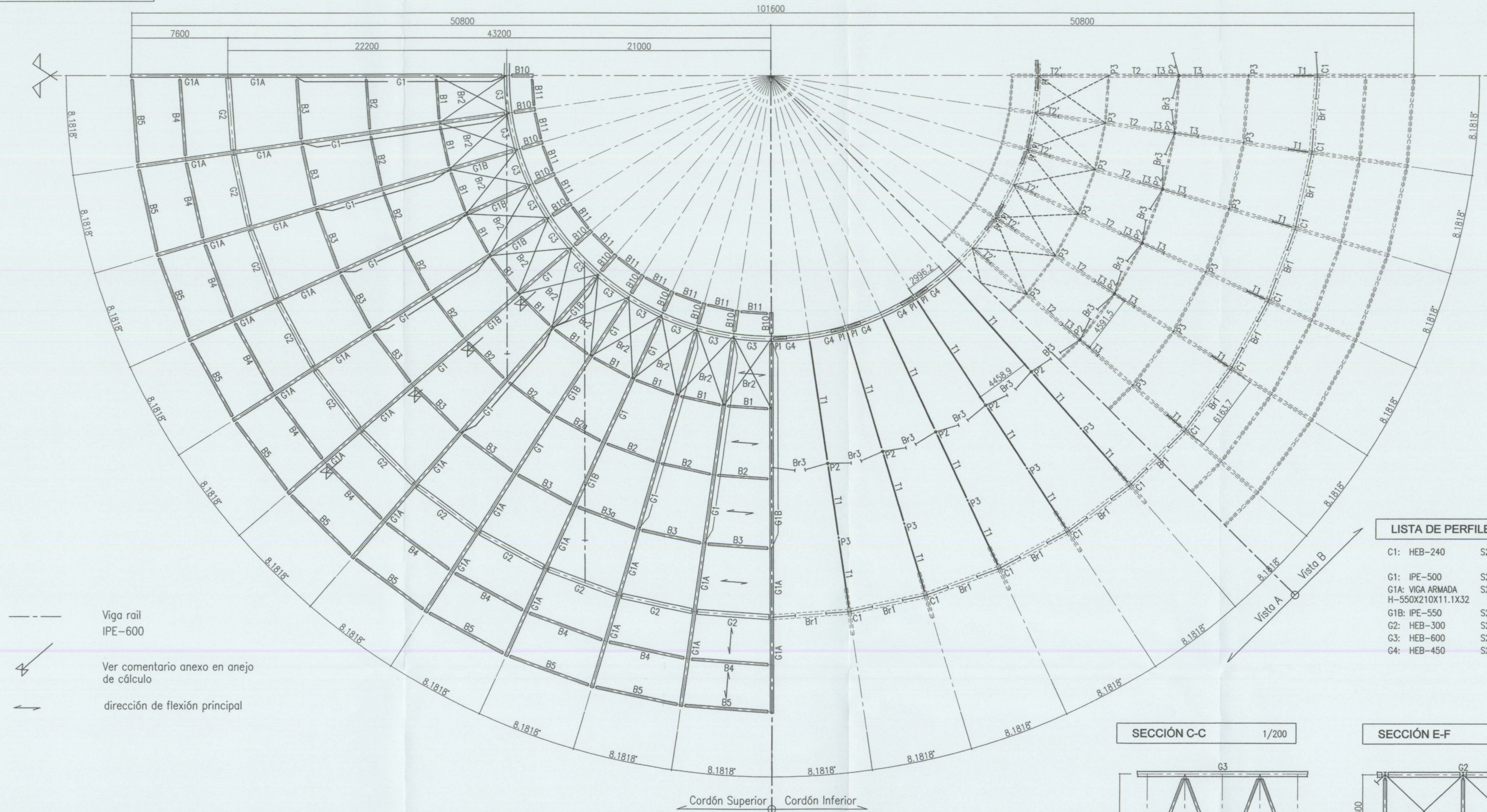
SECCIÓN CUBIERTA FIJA 1/200
