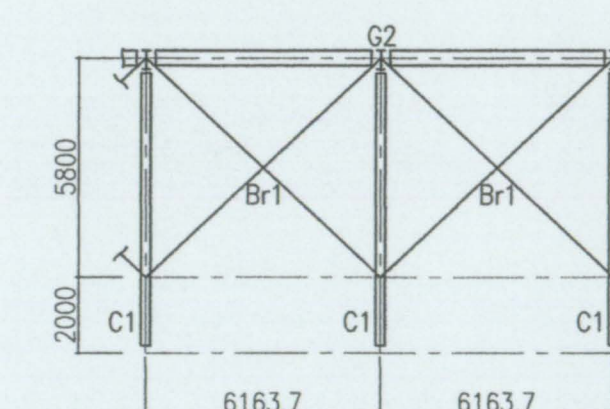
SECCIÓN E-F 1/200
