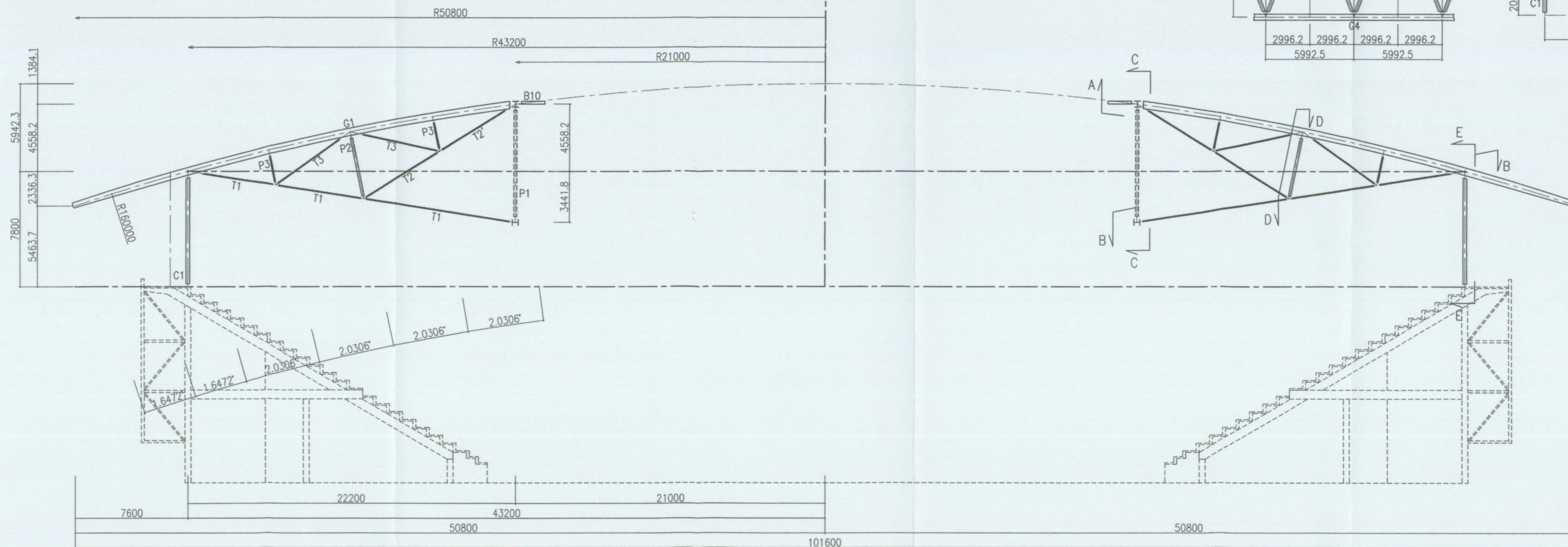
SECCIÓN CUBIERTA FIJA 1/200
